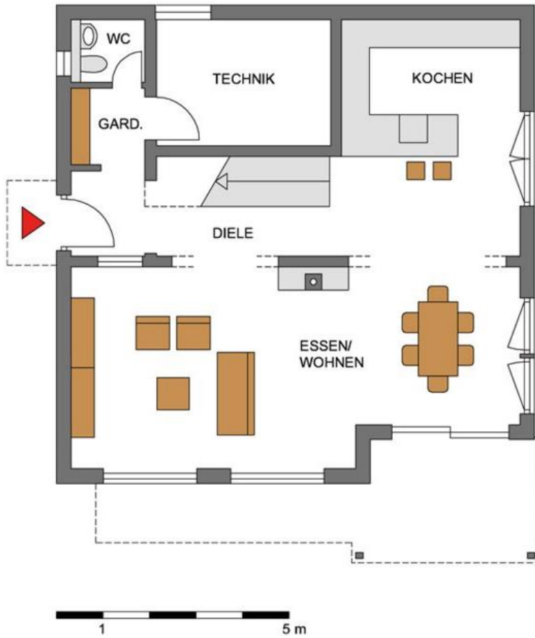
Grundriss Erdgeschoss
