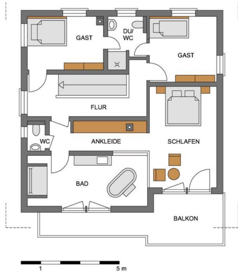
Grundriss Obergeschoss
